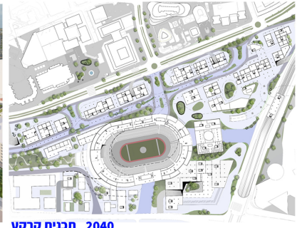
תכנית קרקע 2040
